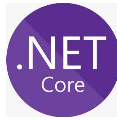
.net core
