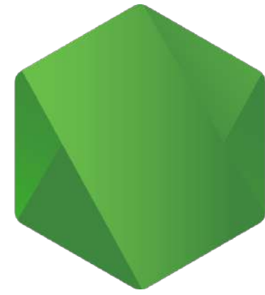
Back-end : Node.js
